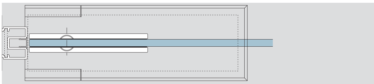
ALEXA PT 35 mit DORMA Universal Eckbeschlägen, Bodentürschließer BTS 75 V ALEXA PT 35 with DORMA Universal patch fitting, floor closer BTS 75 V
