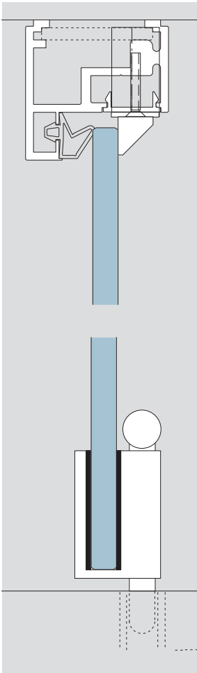
Zargenprofil Frame profile
