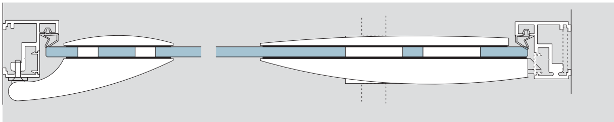
ALEXA AT 44 - mit DORMA ARCOS Studio
