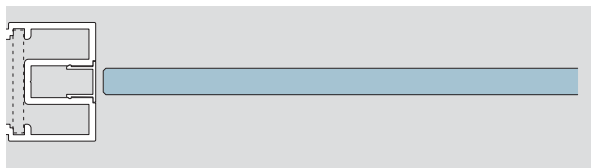
ALEXA PT 35 Zargenprofil mit Clipsprofil ALEXA PT 35 frame profile with cover clip profile
