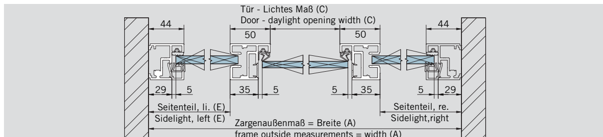
Anschlussrahmen mit AT 44 / Connecting frame with AT 44
