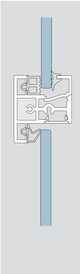
Sprossenprofil Rung profile
