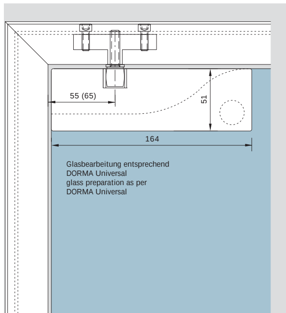
Ansicht DORMA Universal Eckbeschlag oben view DORMA Universal top patch fitting
