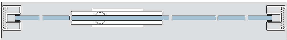
ALEXA PT 35 mit DORMA Universal Eckbeschlägen, Bodendrehlager ALEXA PT 35 with DORMA Universal patch fitting, floor pivot bearing
