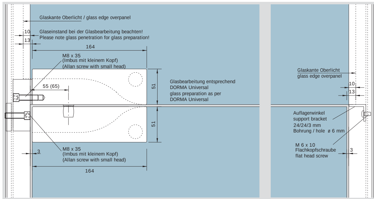
Ansicht DORMA Universal Eckbeschlag view DORMA Universal patch fitting
