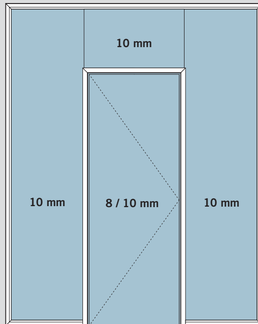
Typ 550 freistehende Zarge
