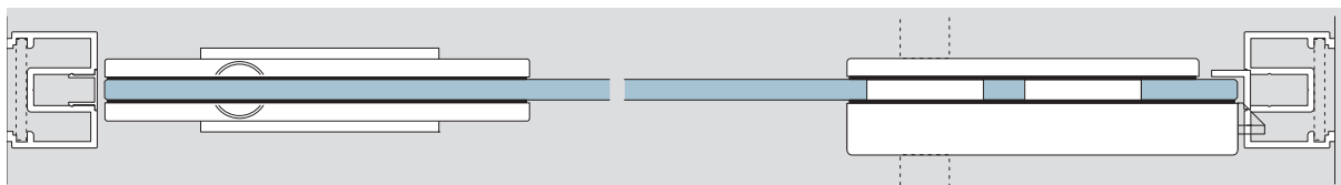
ALEXA PT 35 mit DORMA Universal Eckbeschlägen, Bodendrehlager ALEXA PT 35 with DORMA Universal patch fitting, floor pivot bearing
