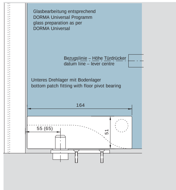
DORMA Universal Eckbeschlag unten, Ansicht view DORMA Universal bottom patch fitting
