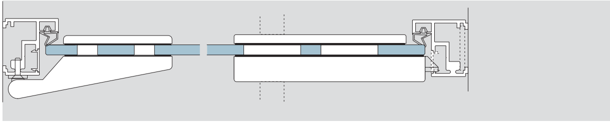
ALEXA AT 44 - mit DORMA Studio (Classic, Rondo)
