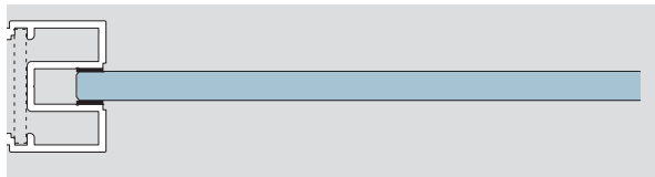
ALEXA PT 35 Zargenprofil mit Glaseinstand ALEXA PT 35 frame profile with glass penetration
