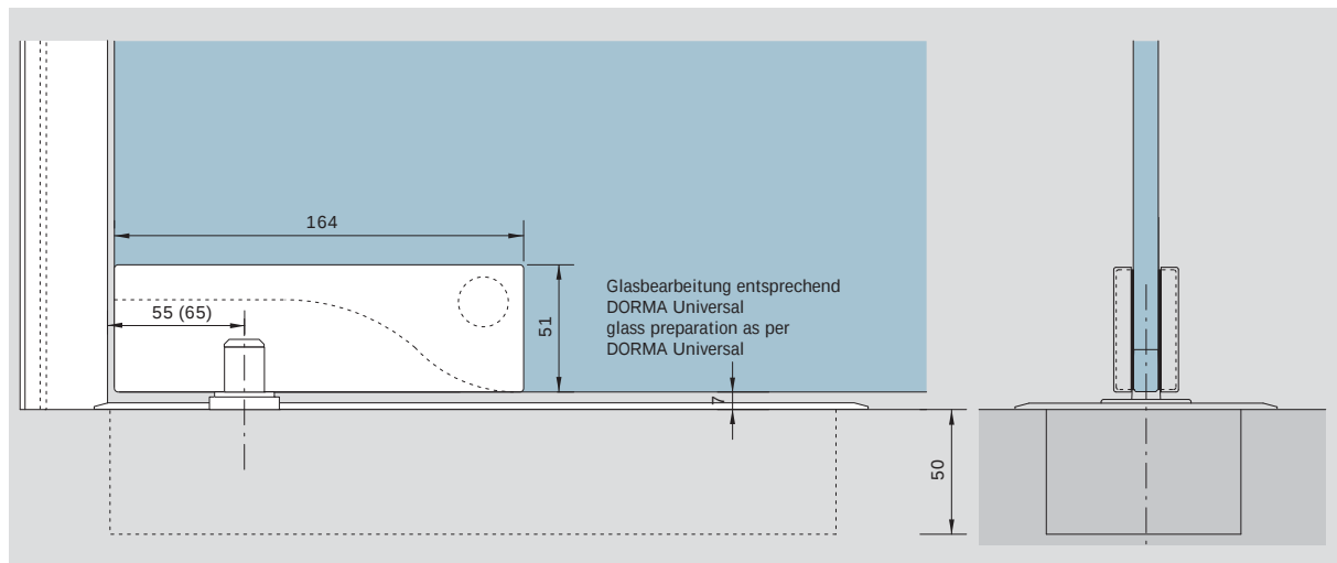
Ansicht DORMA Universal Eckbeschlag, Bodentürschließer view DORMA Universal patch fitting, floor spring
