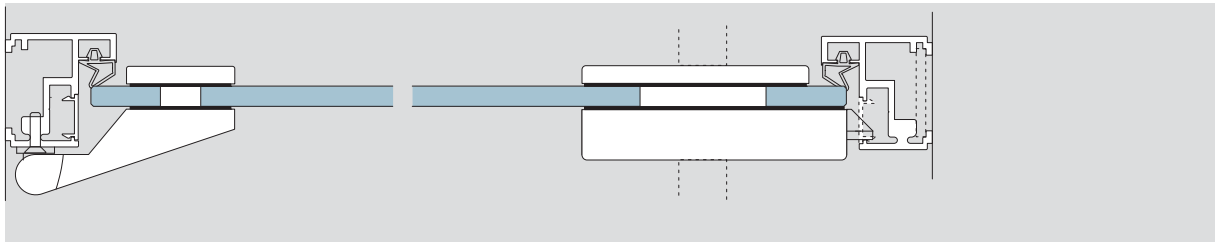
ALEXA AT 44 - mit DORMA Junior (Office, Office Classic)
